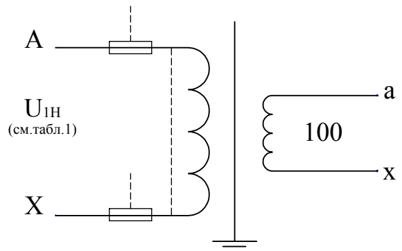
Рис. 3 Принципиальная электрическая схема трансформатора
