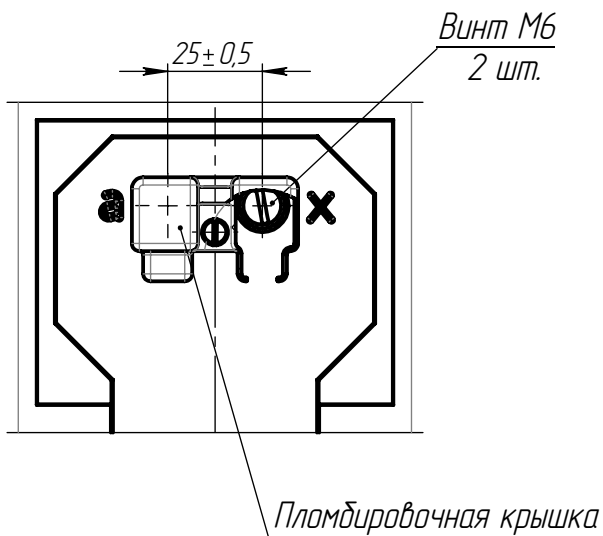
Рис. 2 Клеммник трансформатора напряжения НОЛ-СВЭЛ-6(10)
