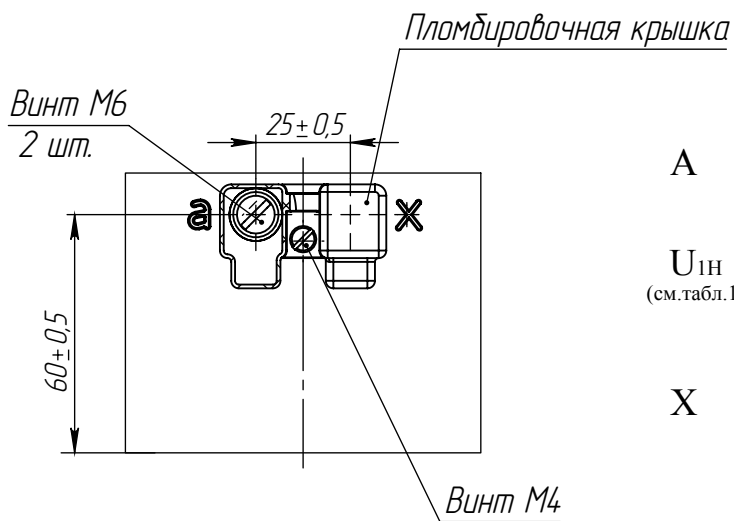
Рис. 2 Клеммник трансформатора напряжения НОЛП-СВЭЛ-6(10)
