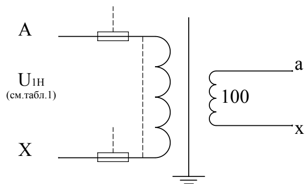
Рис. 3 Принципиальная электрическая схема трансформатора НОЛП-СВЭЛ-6(10)
